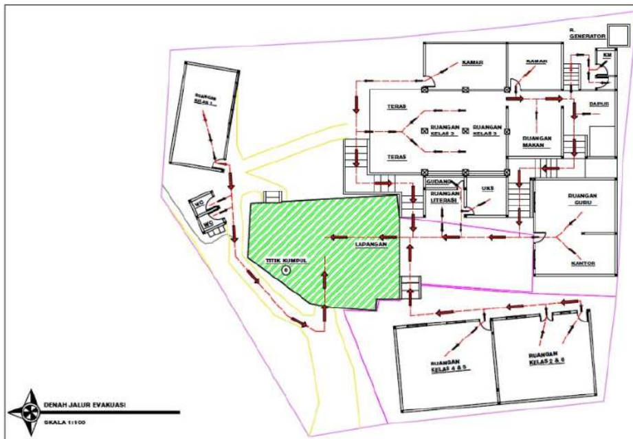
Gambar 6. Arah Jalur Evakuasi
