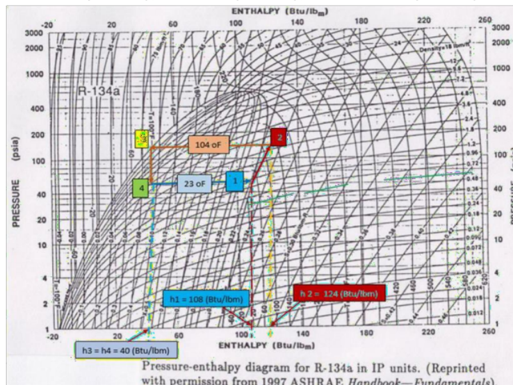
Gambar 1. Diagram P – h untuk refrigerant R-134a
